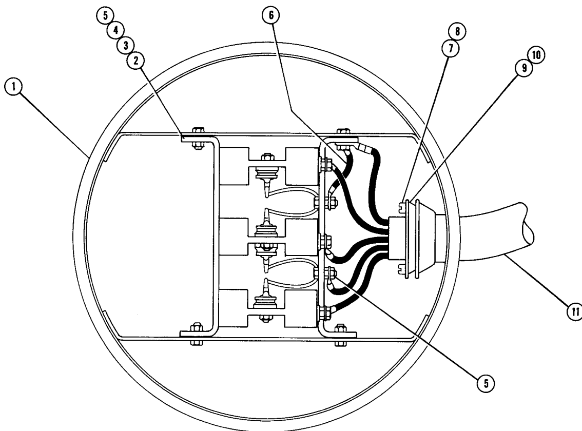
FIG. 8104A RECTIFIER & HOUSING
