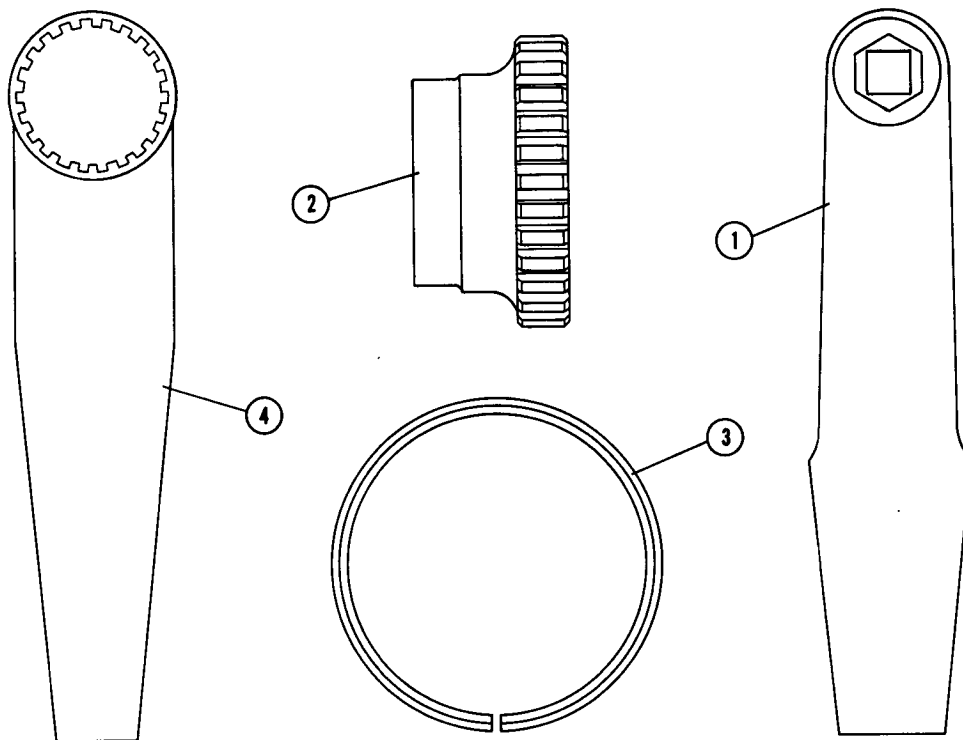
FIG. 6106 A TOOLS
