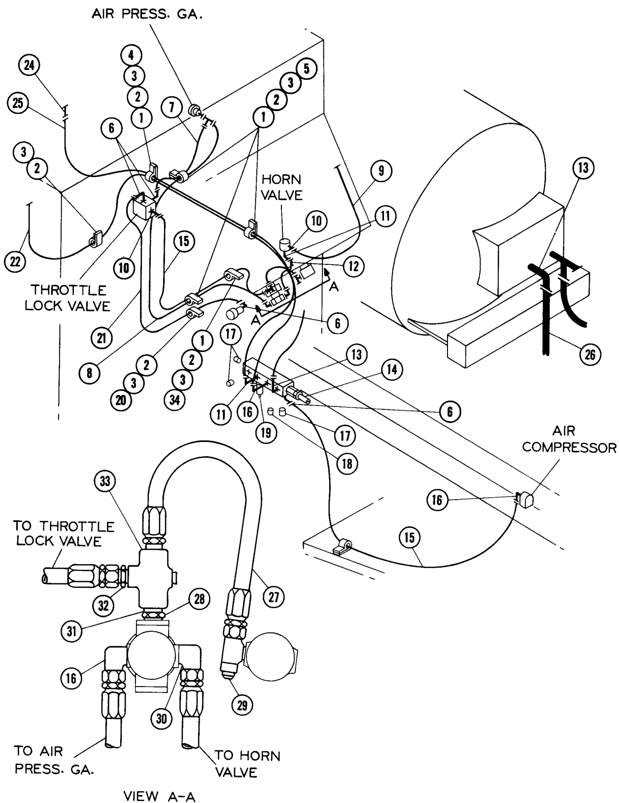
FIG. 6057 PIPING - AIR
