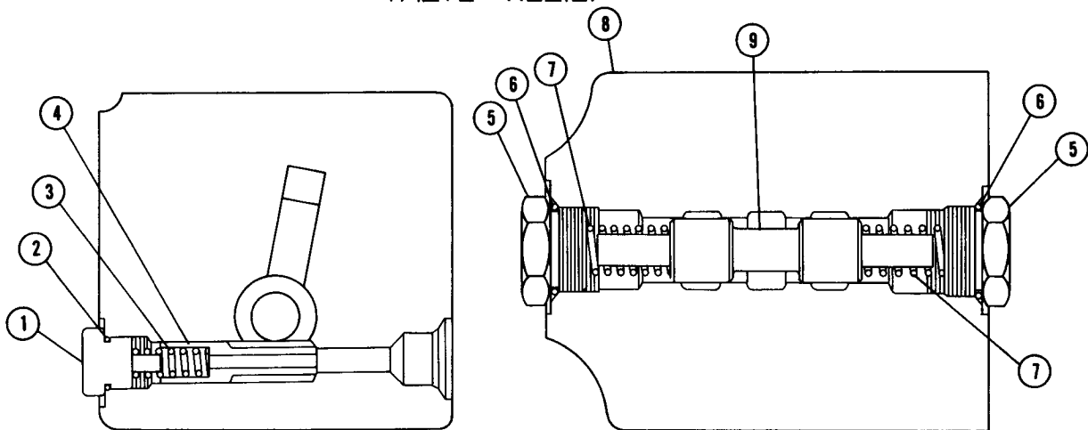
FIG. 5969 B VALVE - RELIEF
