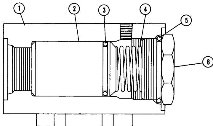
FIG. 5969 A VALVE - CHECK
