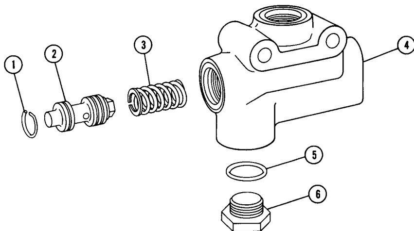
FIG. 5969 B VALVE - RELIEF
