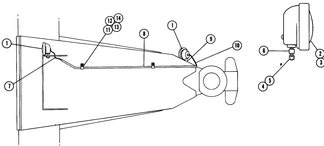
FIG. 6106 B LIGHTS - BLADE & LOAD
