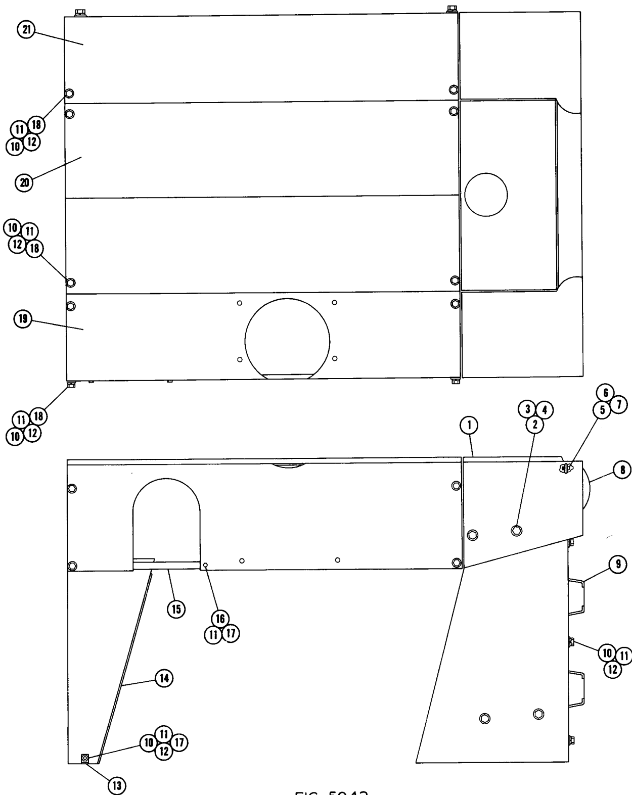
FIG. 5943 GRILL & HOOD
