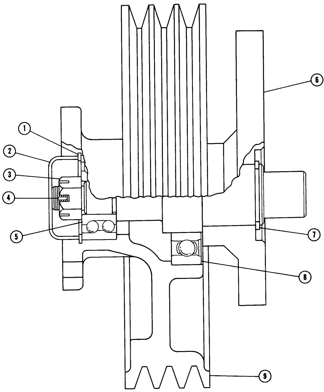
FIG. 5962 FAN BRACKET & HUB
