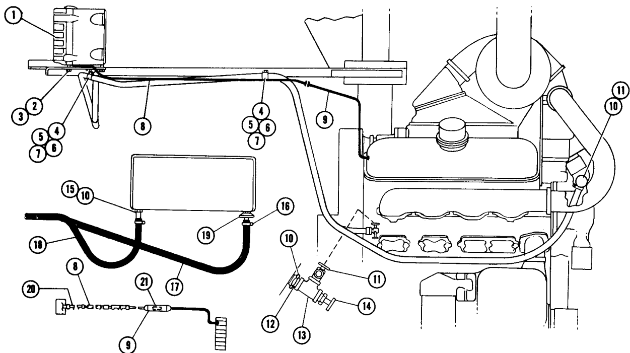
FIG. 6742 A HEATER
