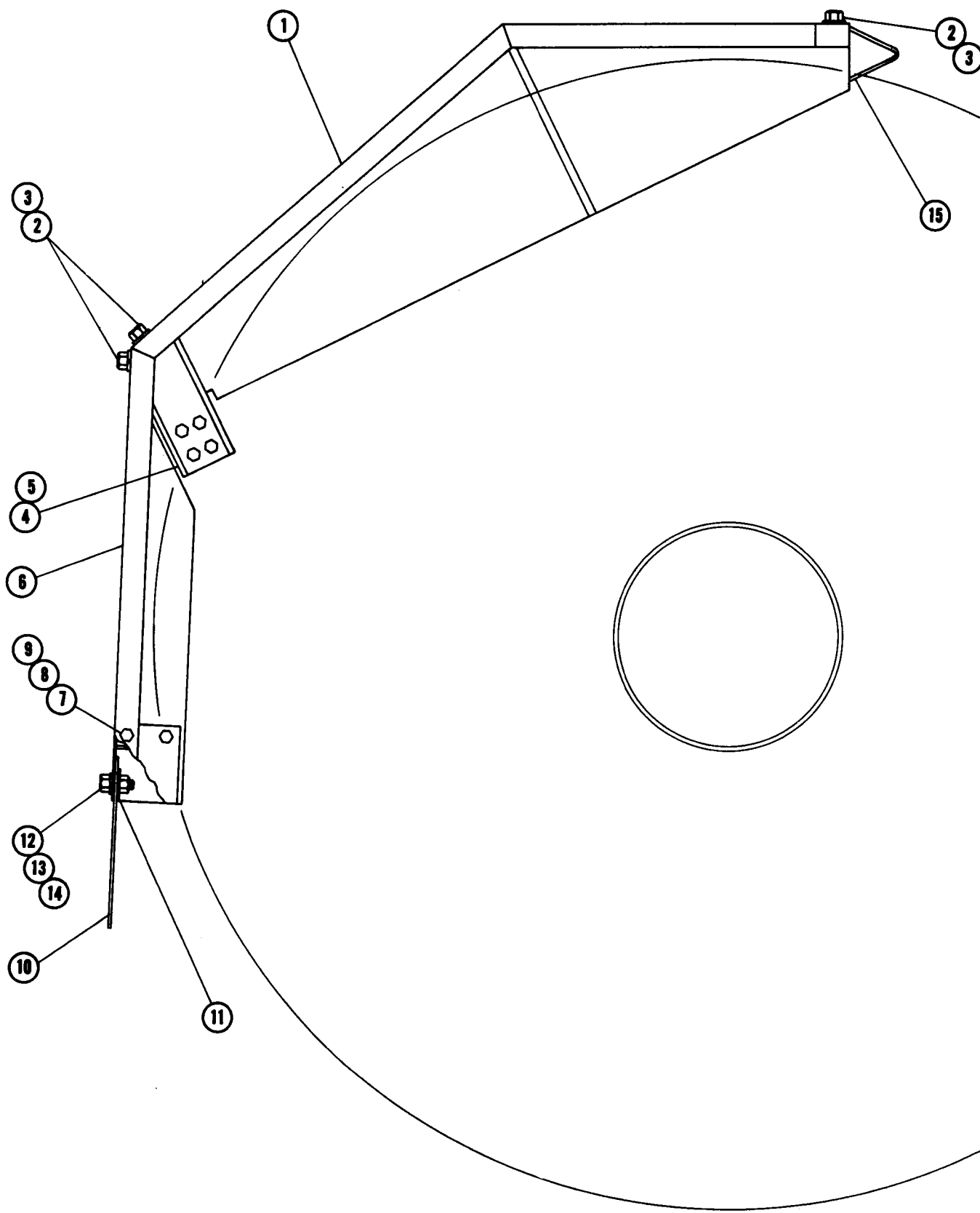
FIG. 7388 FENDERS
