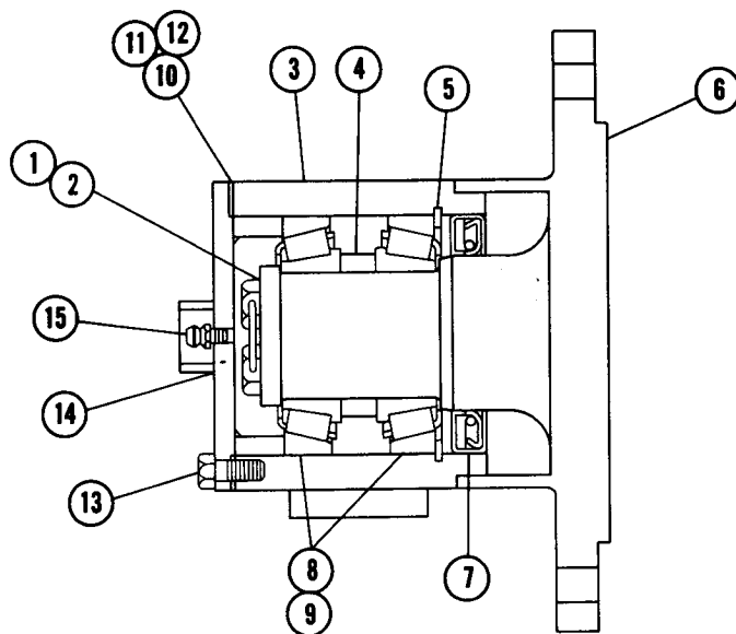
FIG. 6090A HUB & SPINDLE
