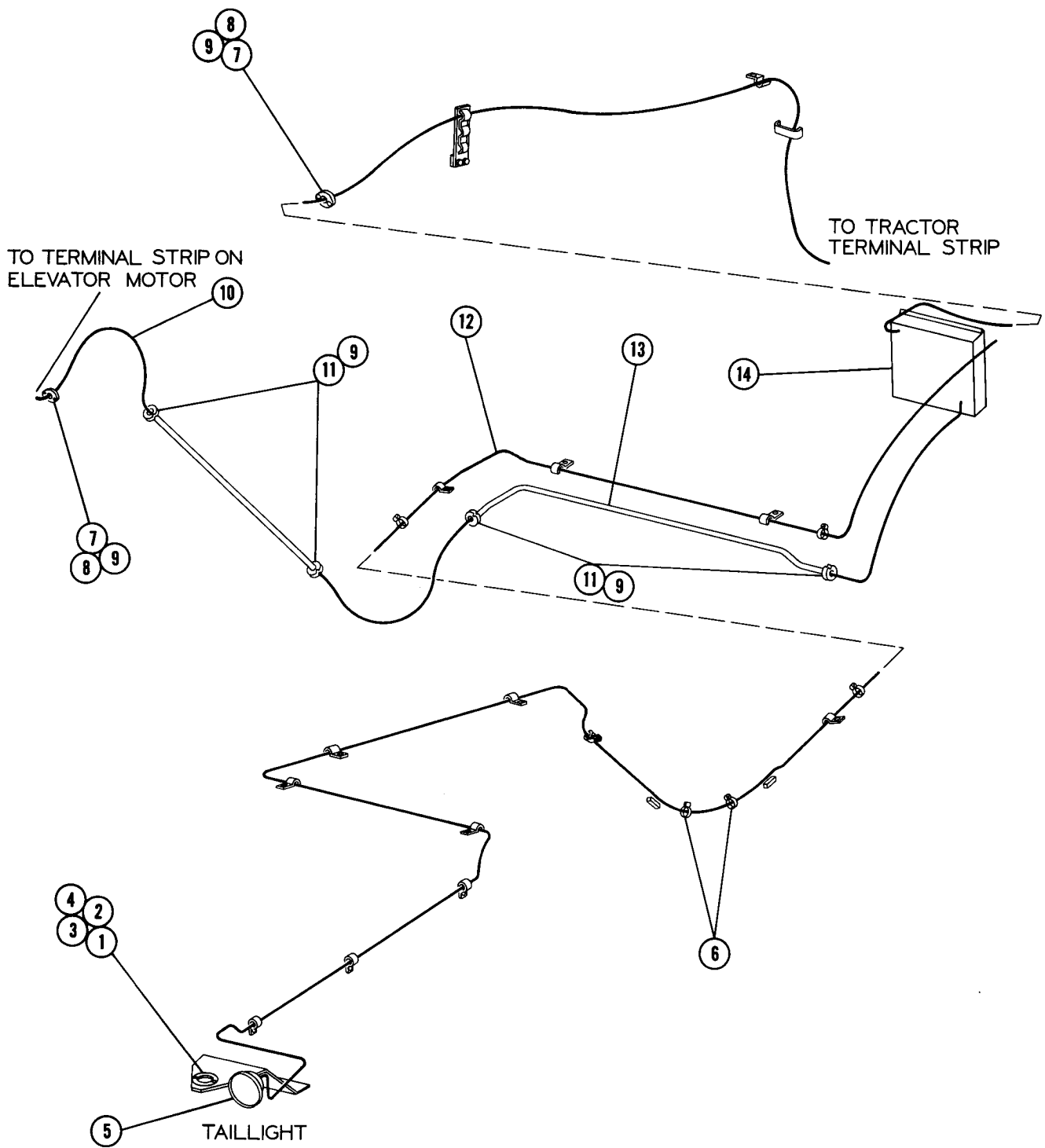
FIG. 6097 WIRING
