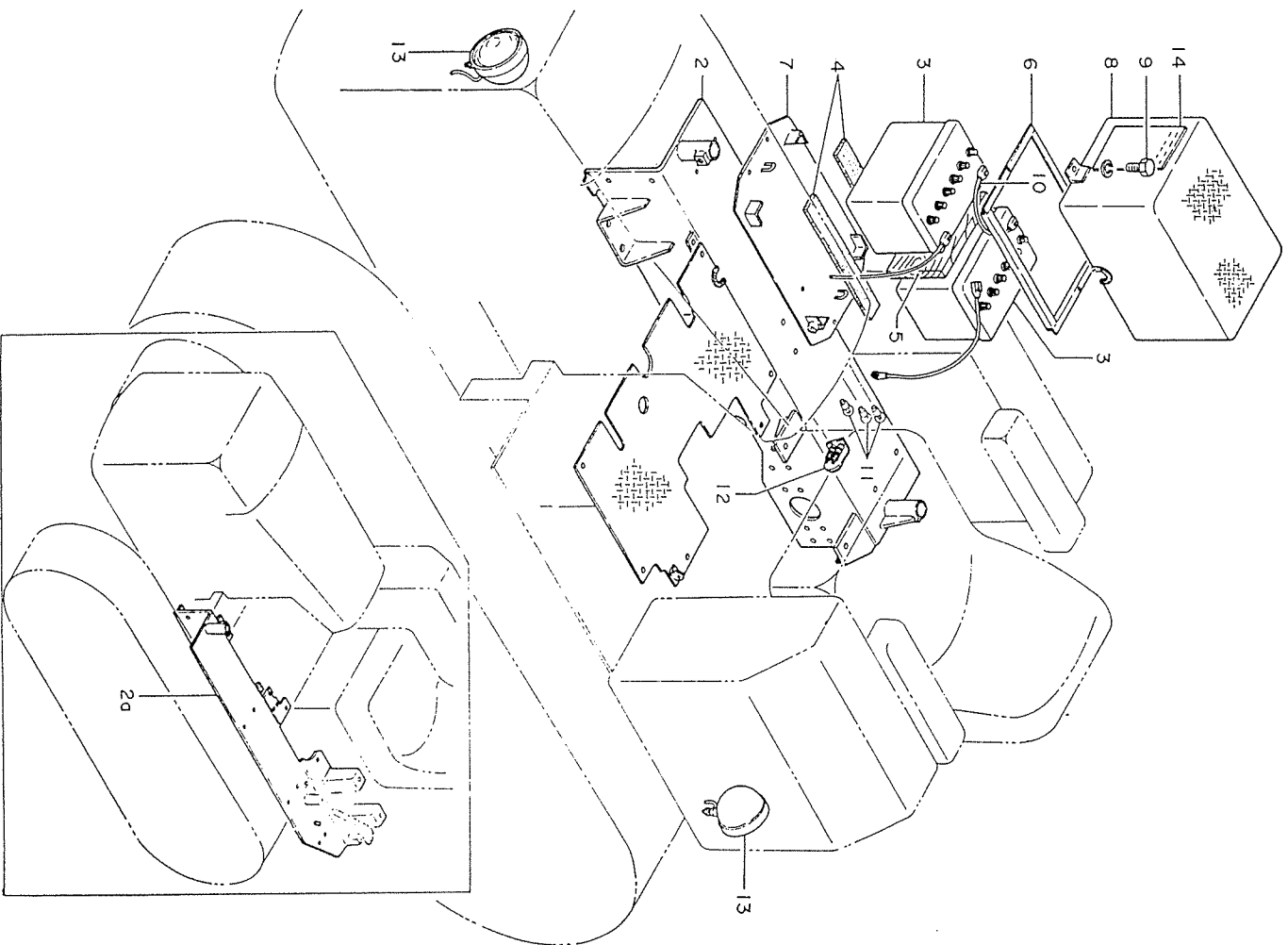
エレクトリックシステム ELECTRIC SYSTEM (NS70.24V) (〜D3d) (OP.) (寒冷地用) (For Cold Local)
