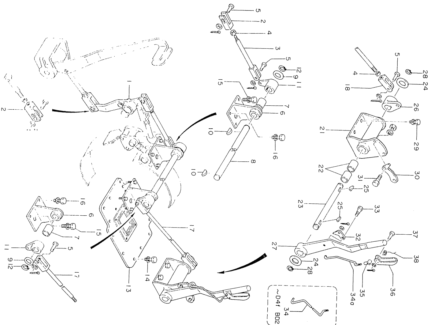
リモート コントロール (バックホーより) REMOTE CONTROLS (From Backhoe) (OP.) ブレーキレバー Brake Lever
