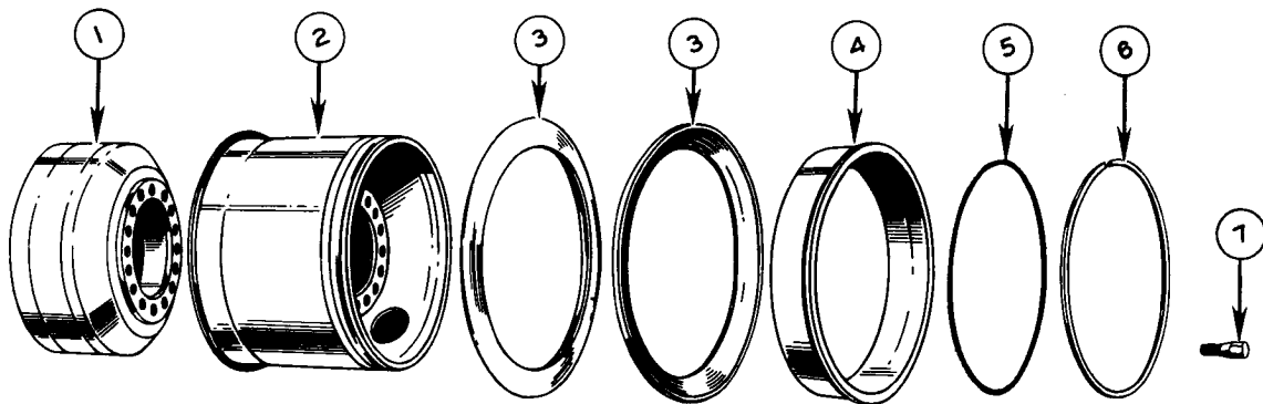
FIG. 1417 C
