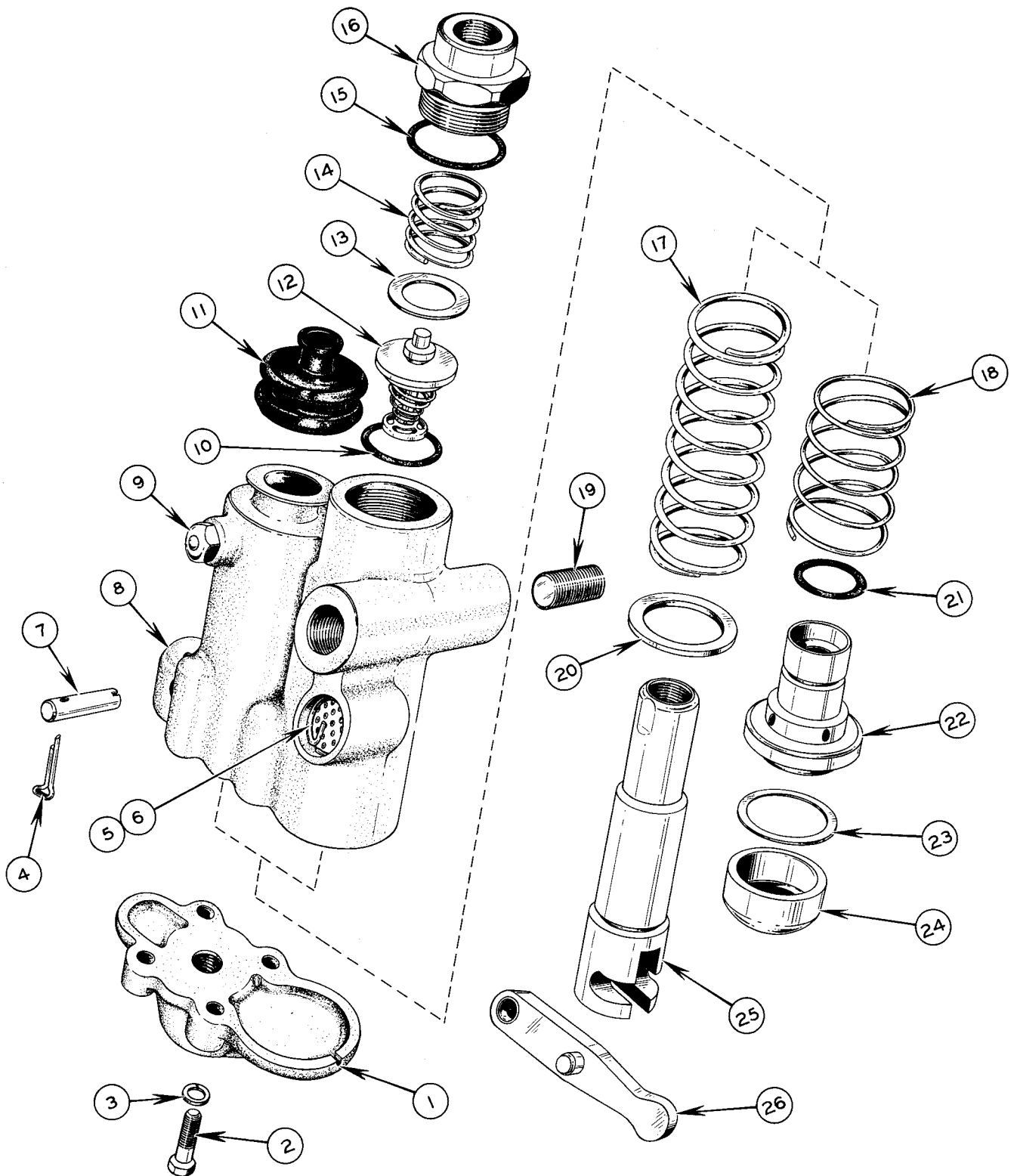
FIG. 944
