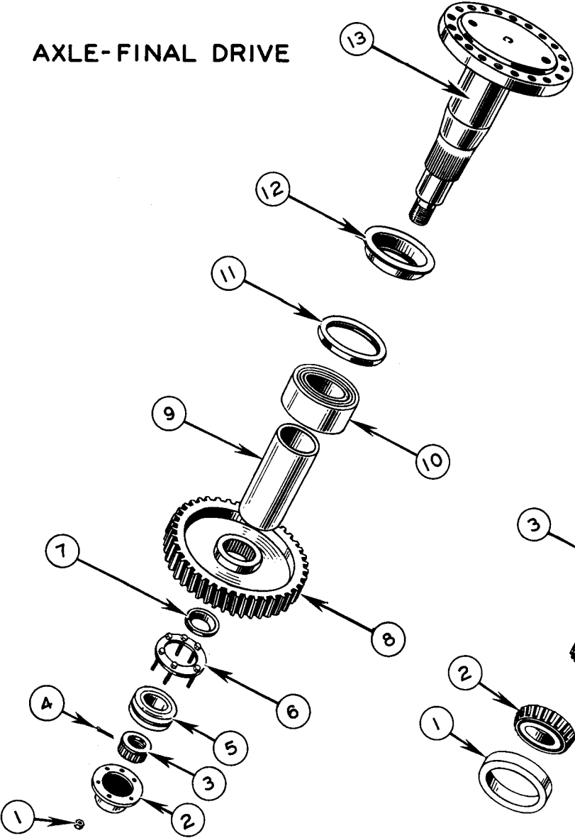
FIG. 2564 A
