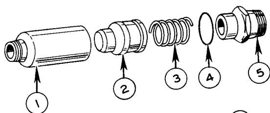
FIG. 2040 A RELIEF VALVE
