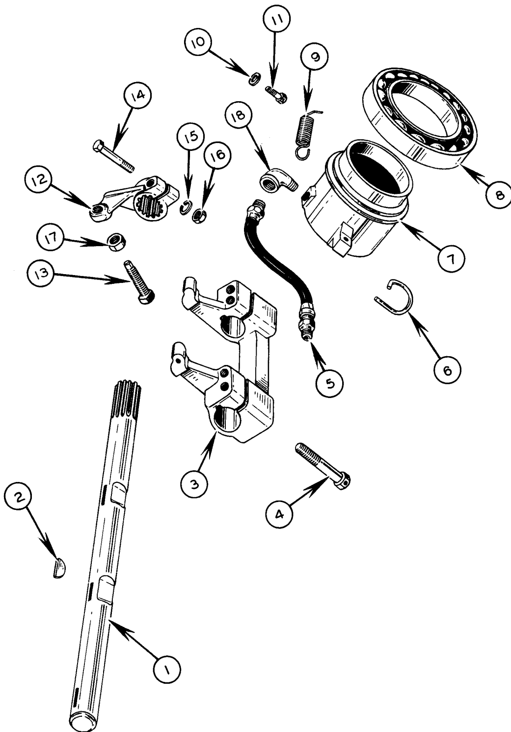
FIG. 1414
