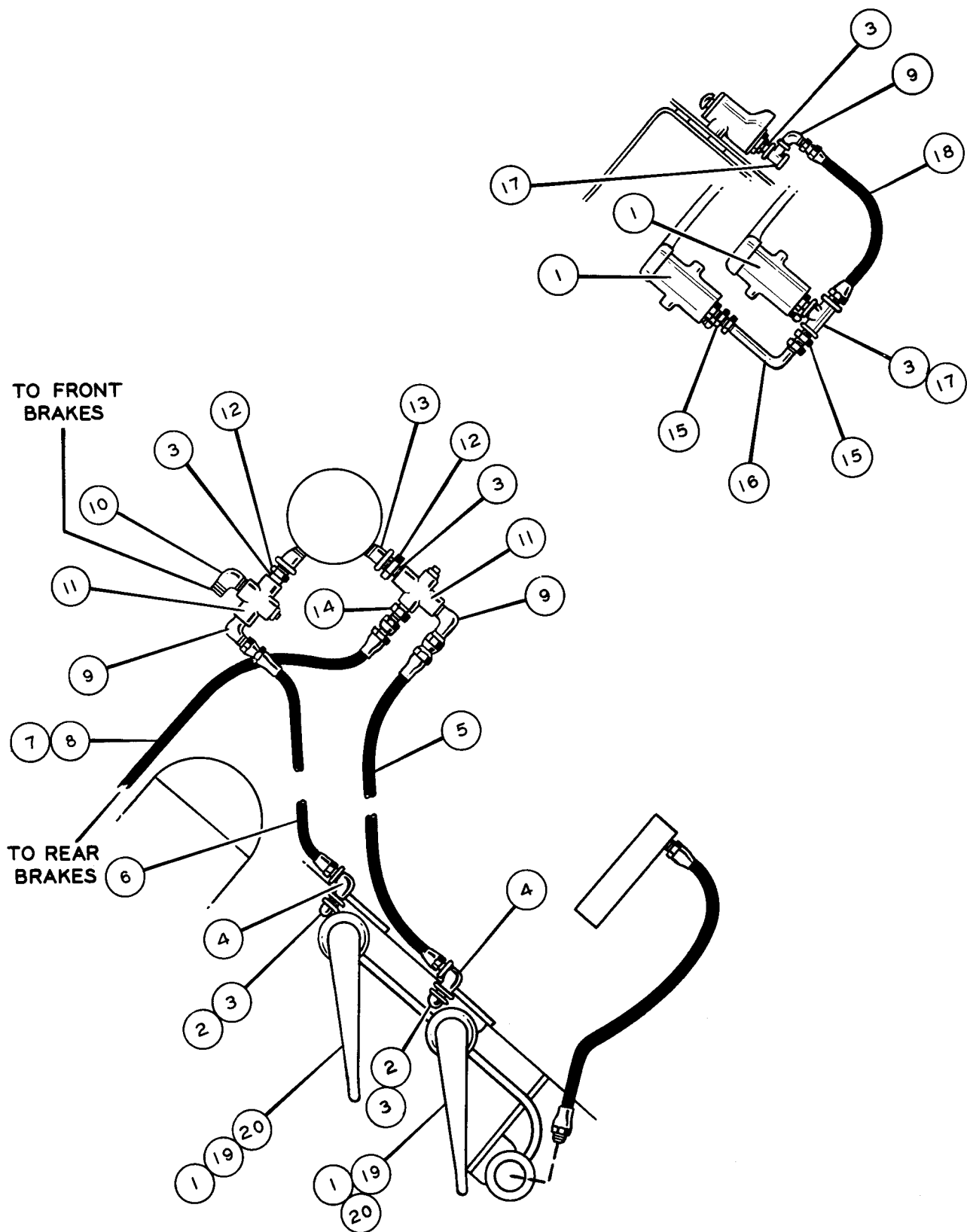
FIG. 2409
