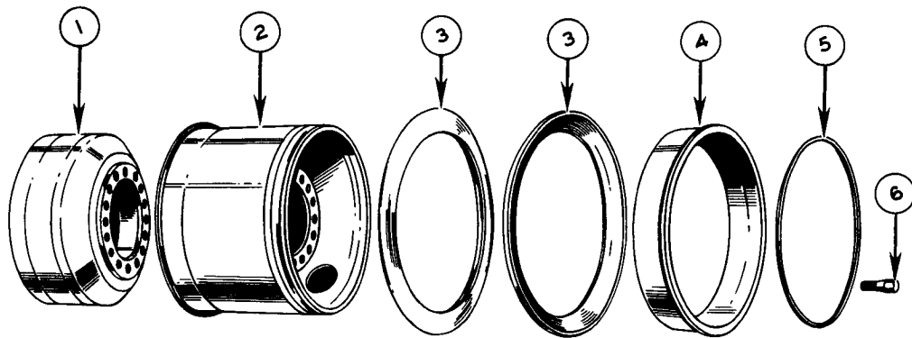
FIG. 1417 C
