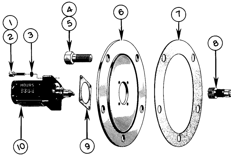
FIG. 1400 A HOUR METER
