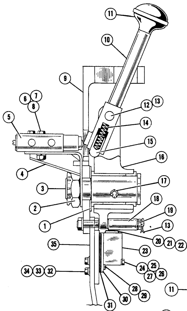
FIG. 3107 A
