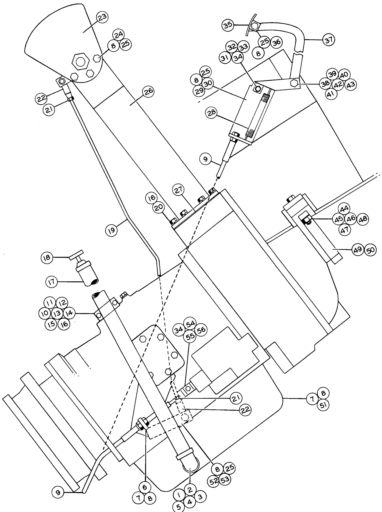
FIG. 2574
