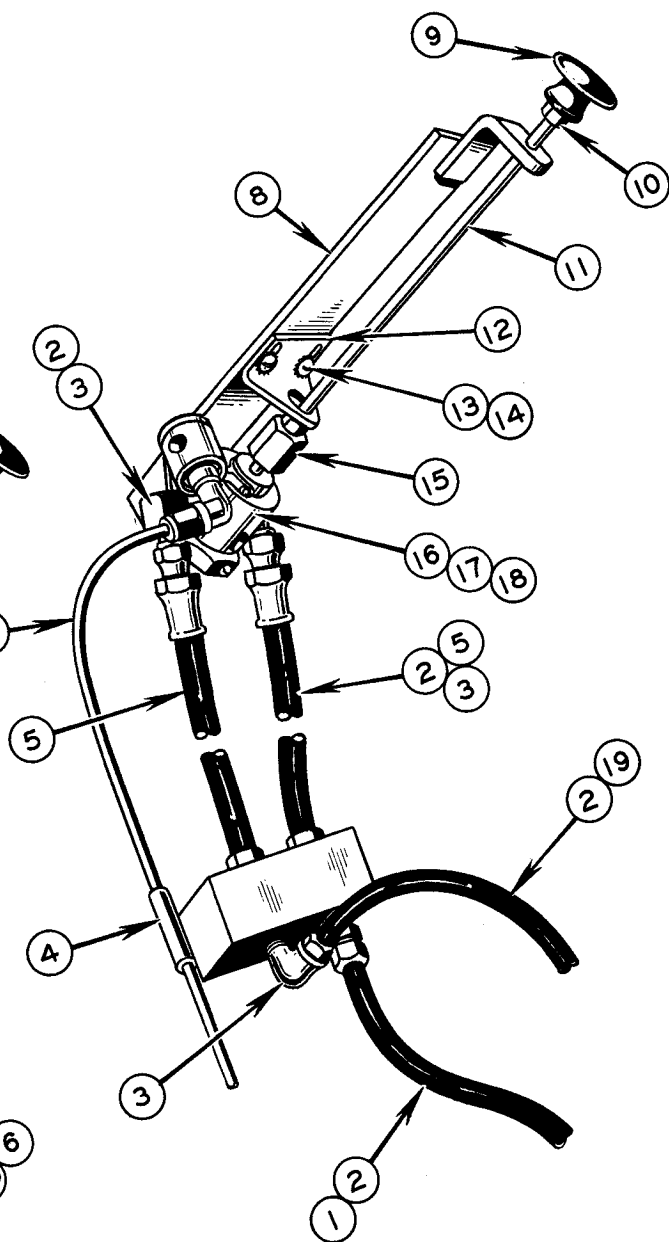
FIG. 1392 B
