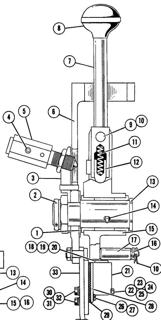
FIG. 3107 B
