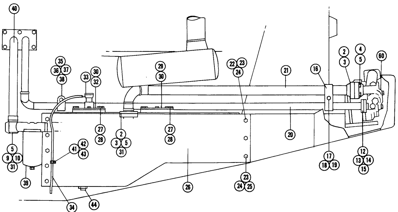
FIG. 3233
