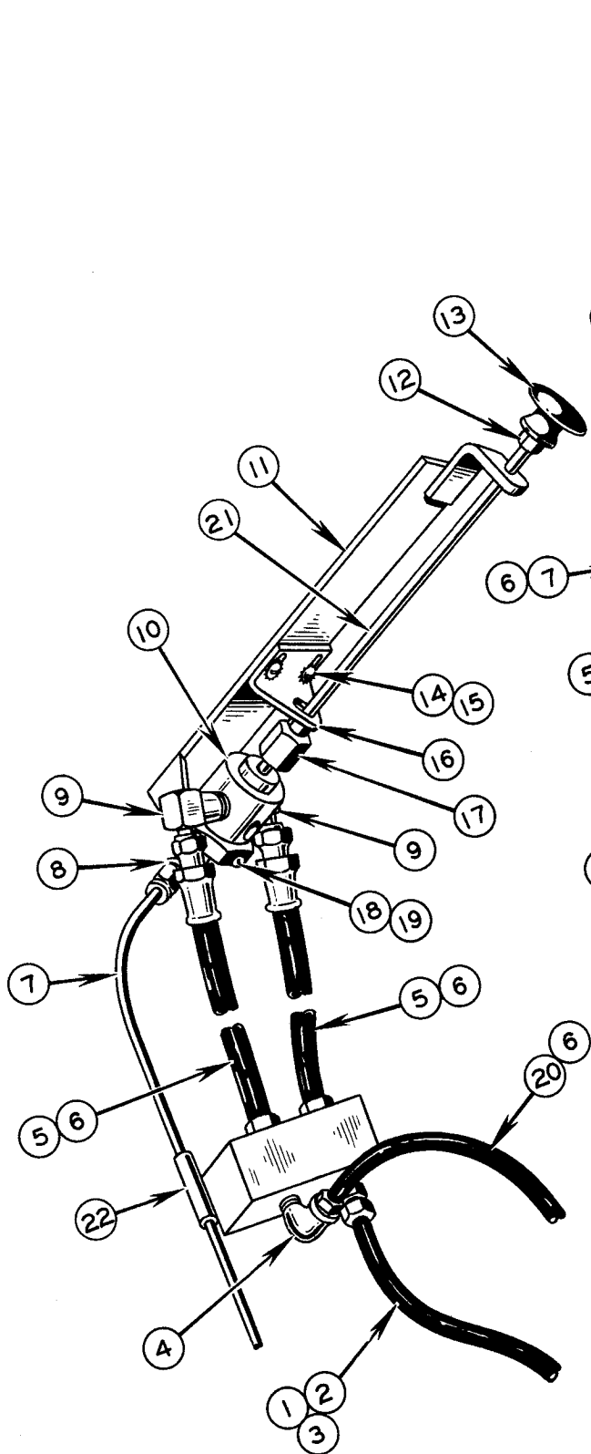
FIG. 1392 A
