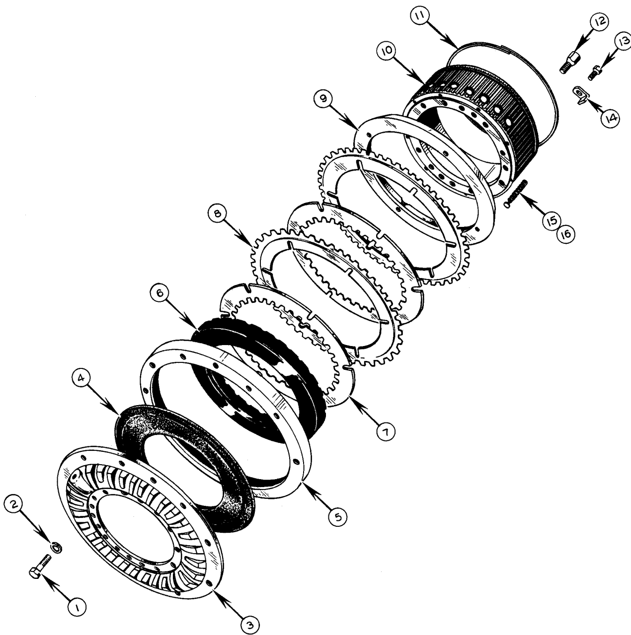
FIG.1234
