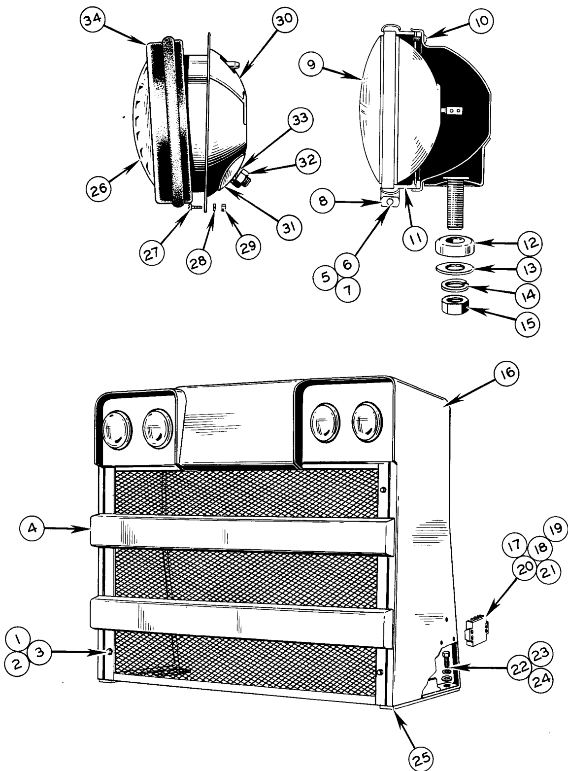
FIG. 1621
