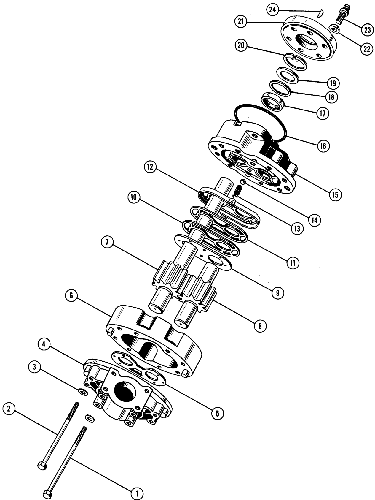
FIG. 3217
