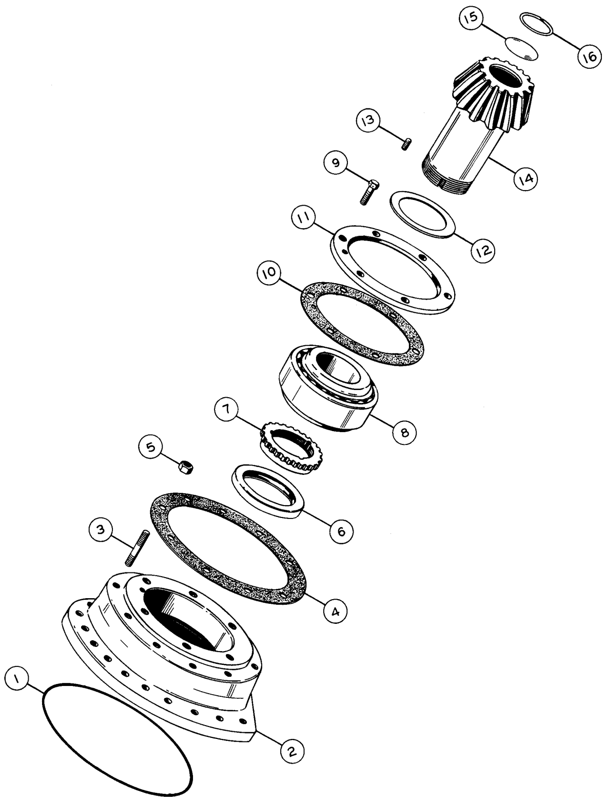
FIG. 2568
