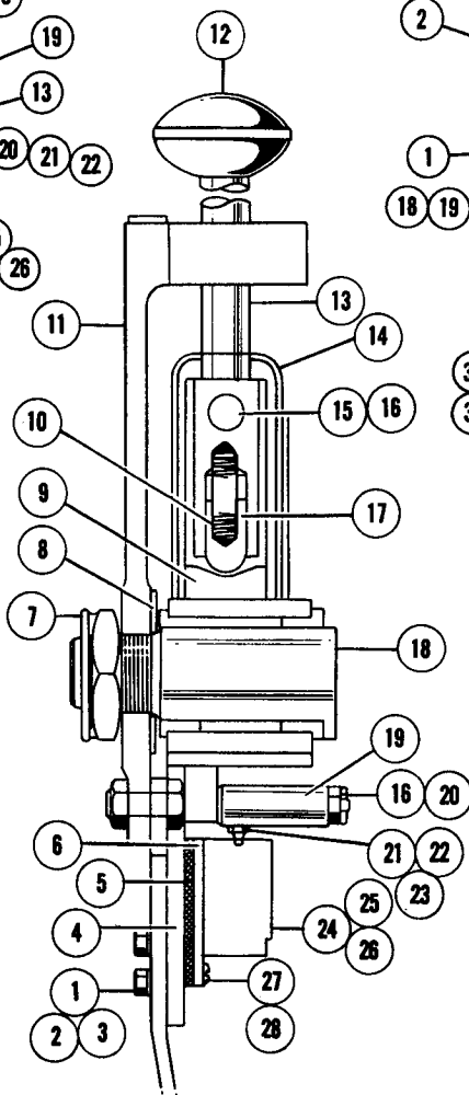
FIG. 3107 C
