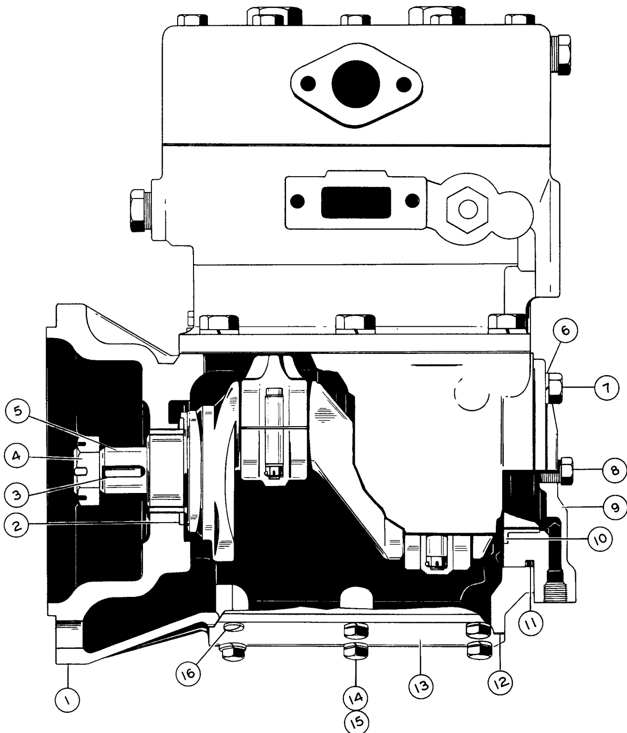
FIG. 2407
