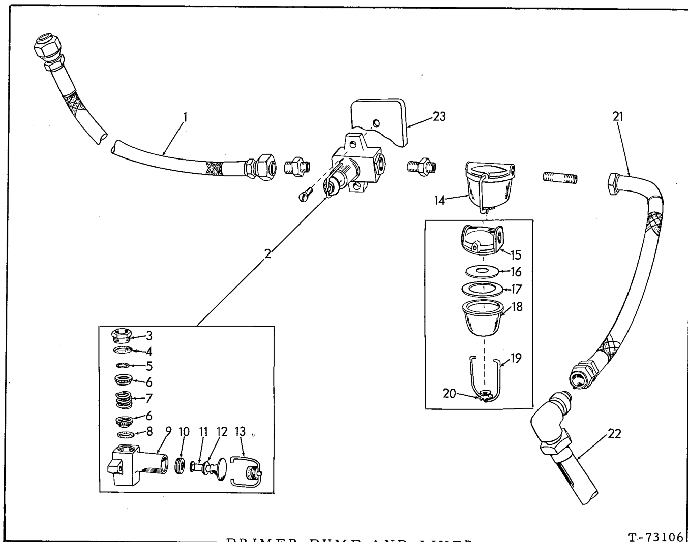
PRIMER PUMP AND LINES
