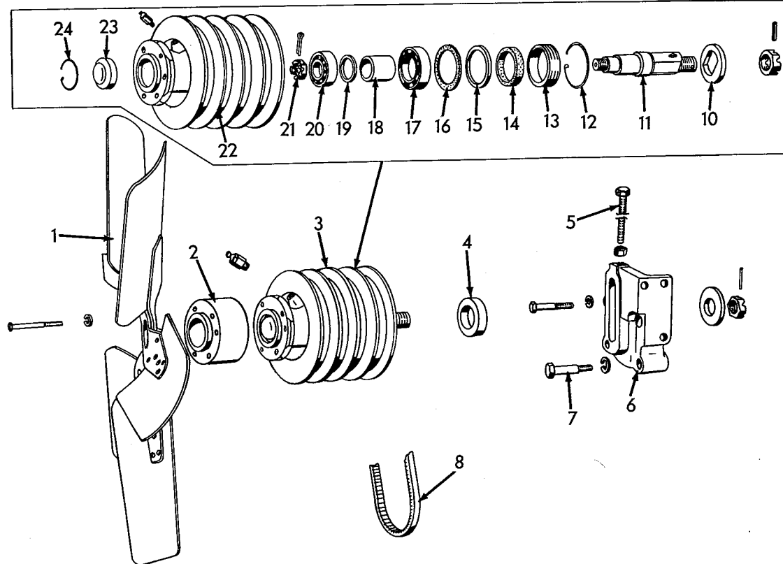
FAN
