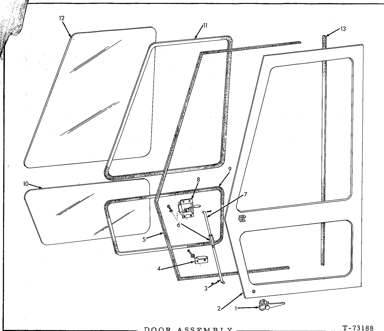
DOOR ASSEMBLY
