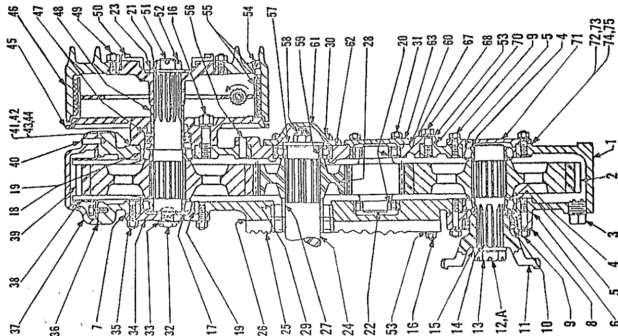
Section A-A
