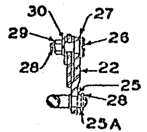
Section D-D
