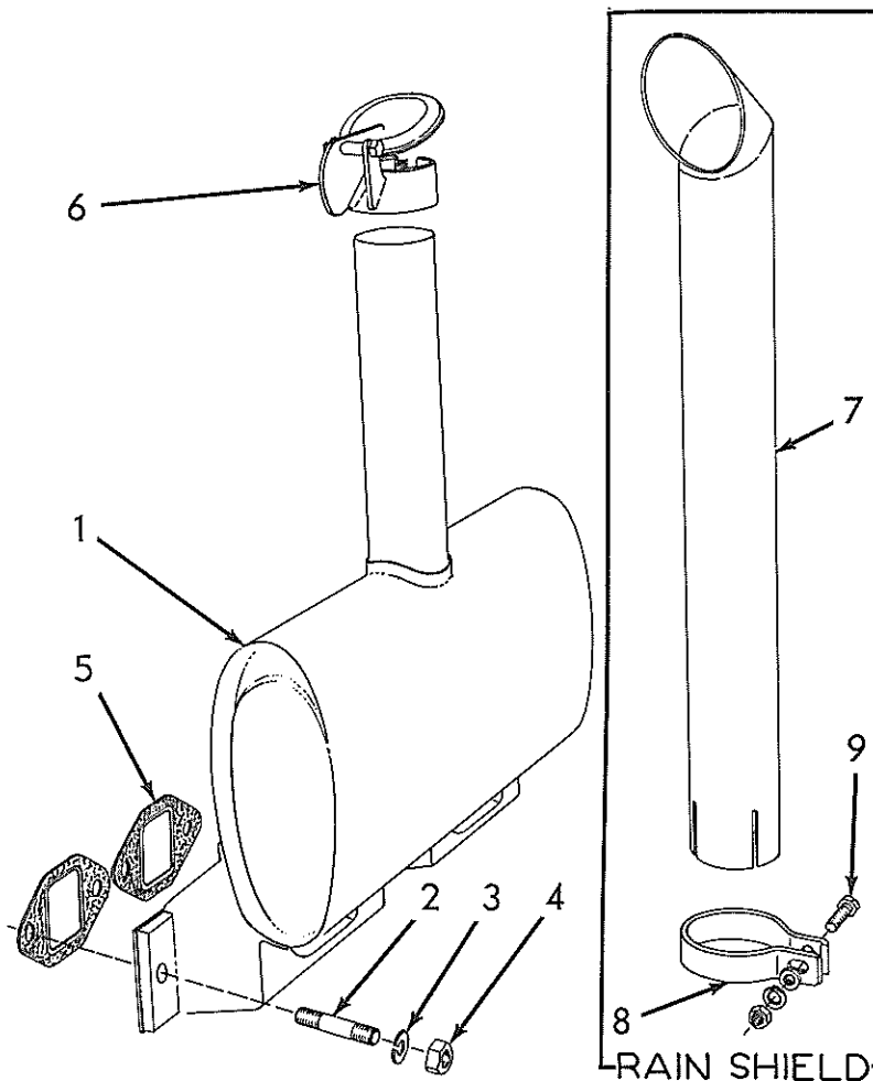
MUFFLER
