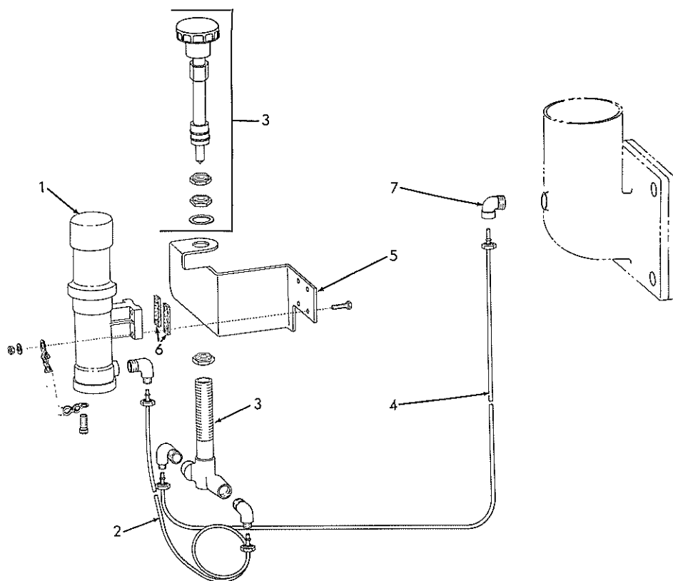
ENGINE PRIMER
