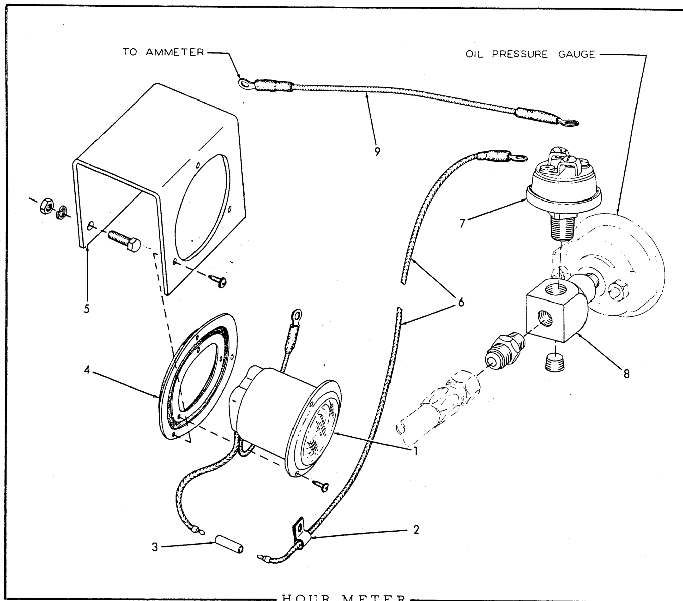
HOUR METER
