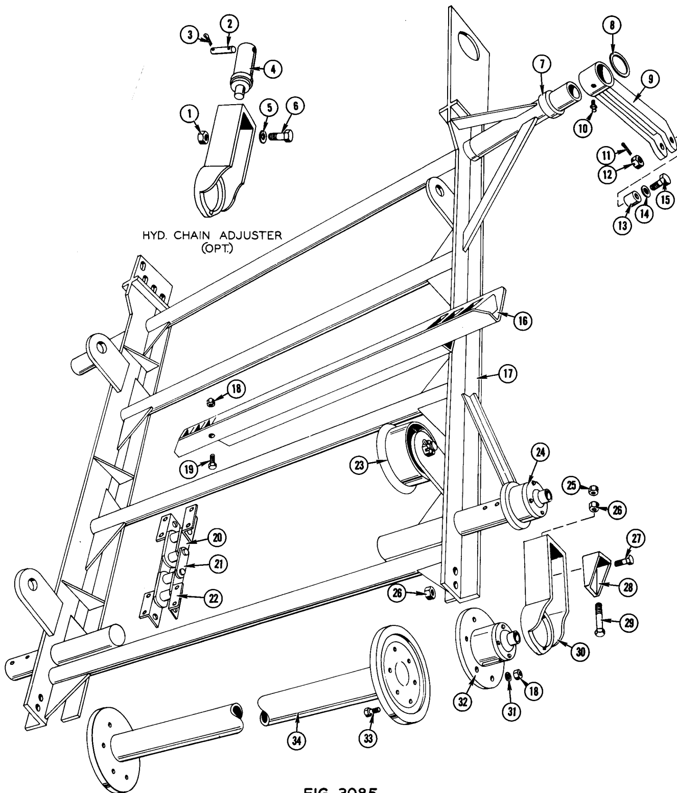
FIG. 3085 ELEVATOR
