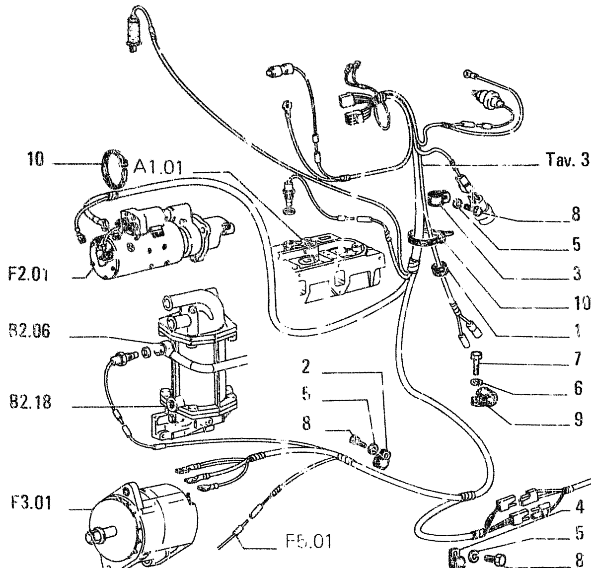
ELECTRICAL SYSTEM IMPIANTO ELETTRICO
