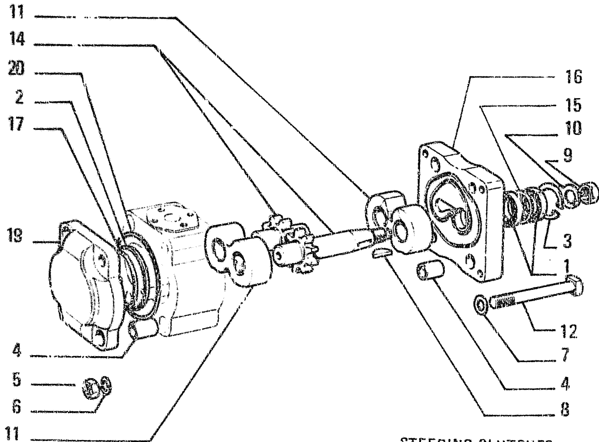
STEERING CLUTCHES FRIZIONI DI STERZO
