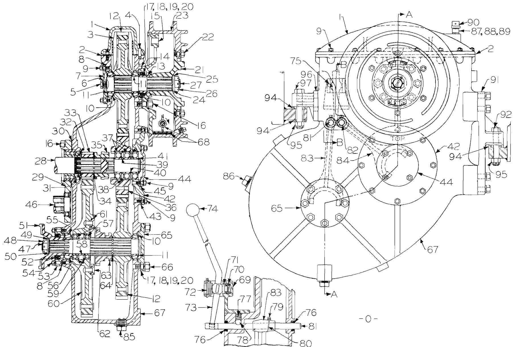
Section A-A
